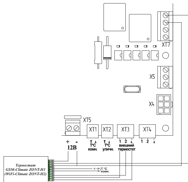
Рисунок 27 Схема подключения термостата GSM-Climate, WiFi-Climate
