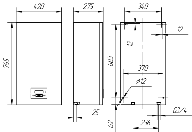
Рисунок 11. Габаритные и присоединительные размеры прибора.
