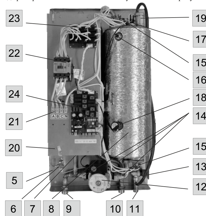
Рисунок 3 Прибор EXPERT-S со снятыми лицевой панелью и кожухом
