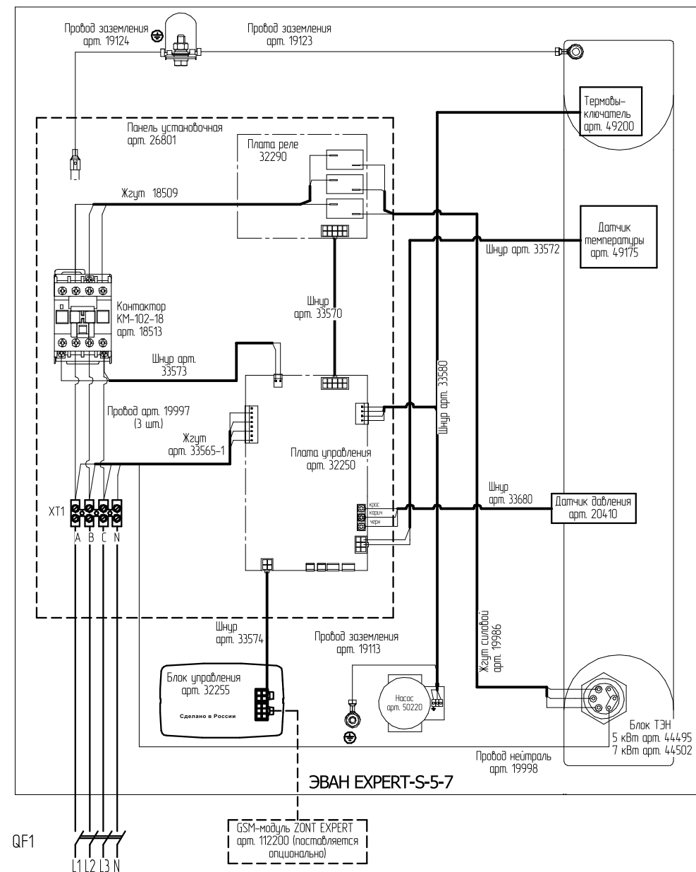
Рис. 13 Схема подключения ЭВАН EXPERT-S-5...7 к сети 380 В
