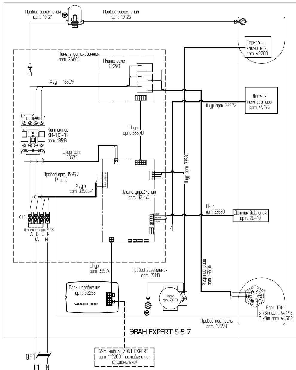
Рис. 12 Схема подключения ЭВАН EXPERT-S-5...7 к сети 220 В
